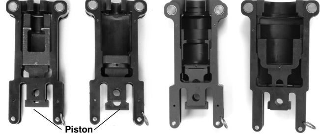
Figure 1 – Gabarits de sertissage Ø 1/4, 1/2, 7/8, et 1 1/8 pouces
